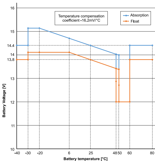
Temperatuurgecompenseerde laadgrafiek
