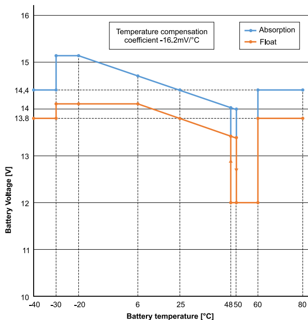
Temperatuurcompenseerde laadgrafiek
