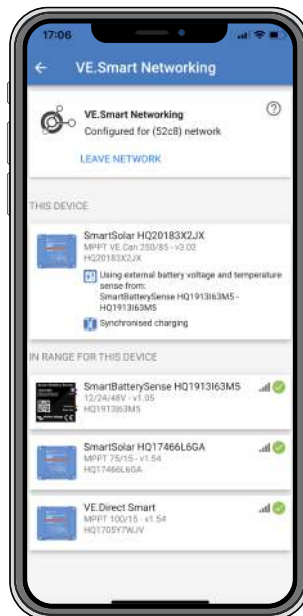
Voorbeeld van een VE.Smart-netwerk
