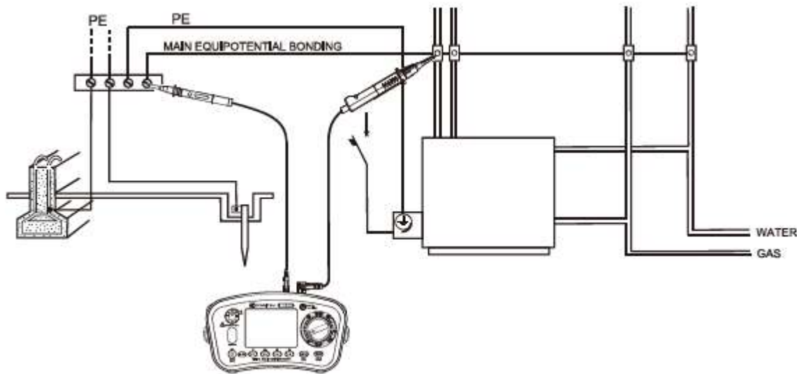
Figuur 8-4 Voorbeeld van een continuïteitstest voor de hoofduitrustingspotentiaalvereffening.
