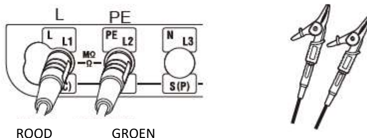
Figuur 10-18 voor L-PE 2-draads test
