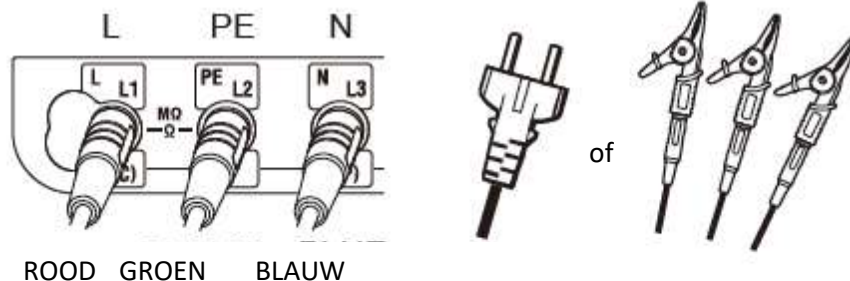
Figuur 10-17 voor L-PE 3-draads test
